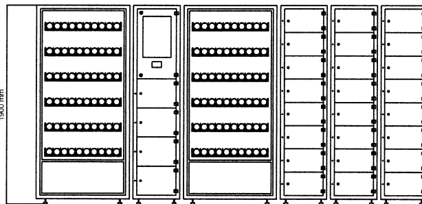
Double distributeur automatique de consommables (DAC) à vrilles, un module de dialogue utilisateur, armoires de casiers complémentaires (distribution de consommables, outillages, consignés)
