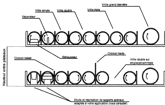
40 modèles de vrilles pour s'adapter aux diverses tailles (profondeur) des articles distribués
