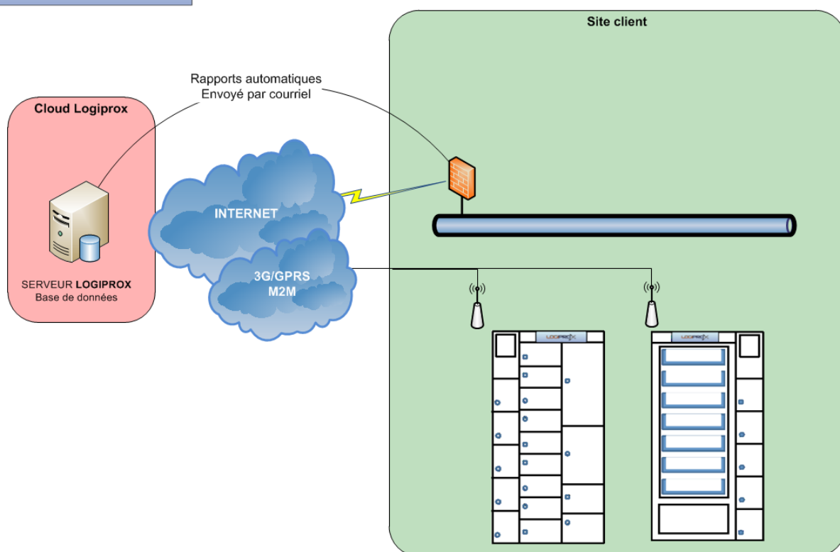
Schéma réseau 3G
