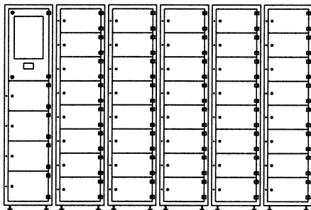
Module de dialogue utilisateur, armoires de casiers complémentaires (distribution de consommables, outillages, consignés)
