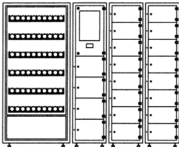
Distributeur automatique de consommables (DAC) à vrilles et son module de dialogue utilisateur, armoires de casiers complémentaires (distribution de consommables, outillage, consignés)
