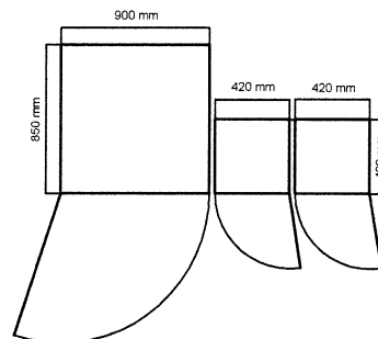
Encombrement au sol et zones d'ouverture des portes (ajouter espace de passage pour les utilisateurs)
